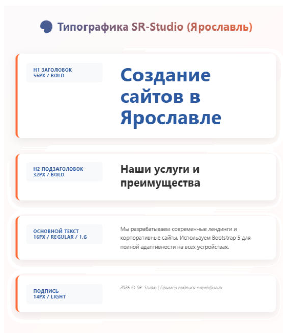
Рисунок 9 Сетка типографики.
